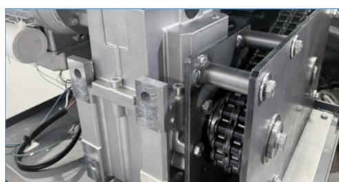
Il modello Kobra DIGITAL-PRO è equipaggiato con il motoriduttore in acciaio "Titan-Colossus" in grado di distruggere grandi quantità di: SSD (anche con case in metallo), smartphone, schede SIM, chiavette USB, chip di memorie flash IC, carte di credito con chip, schede elettroniche, CD/DVD.
