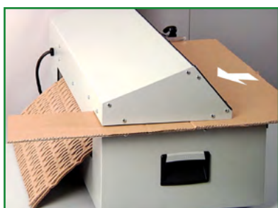
Facile da usare: larghezza dell'entrata cartone regolabile. Taglia in automatico cartoni di larghezza superiore alla luce d'entrata.
