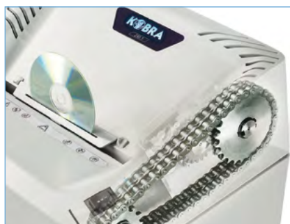
Robusta trasmissione a catena con ingranaggi in acciaio. Flap di sicurezza.
