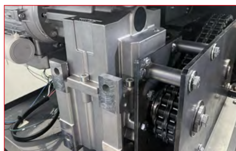
Il modello Kobra GAMBLER è equipaggiato con il motoriduttore in acciaio "Titan-Colossus" in grado di distruggere grandi quantità di materiali sensibili da gioco come dadi, fiches, gettoni e carte da gioco.
